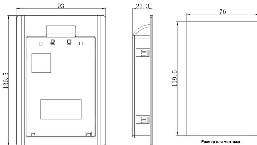
Рис. 1-7 Габаритные размеры панели управления
