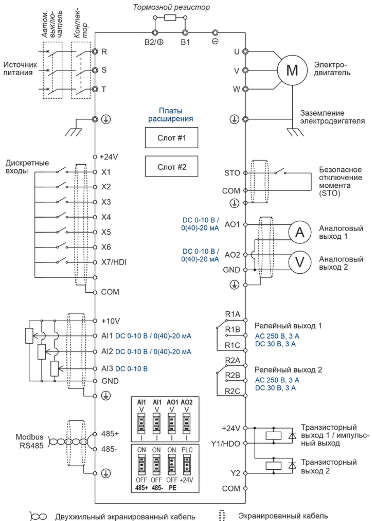
Рис. 2-4 Стандартная схема подключения
