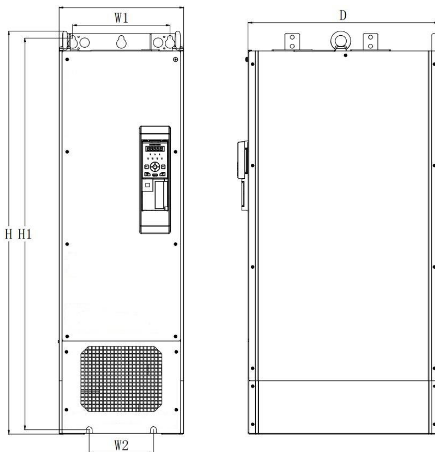
Рис. 1-6 Установочные размеры IMD224U43E~IMD404U43E (220кВт~450кВт)
